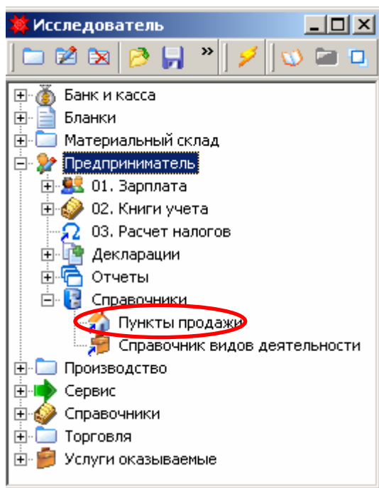
Рис. 1. Окно исследователя
